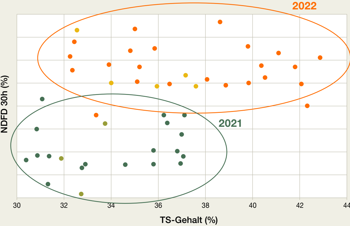
Grafik 1: NDFD 30h – Vergleich der Jahre 2021 + 2022, Mittelwerte von 3 Orten (n = 12; SüdNds, Niederrhein, Nordbaden), TS-Gehalt x NDFD 30h
