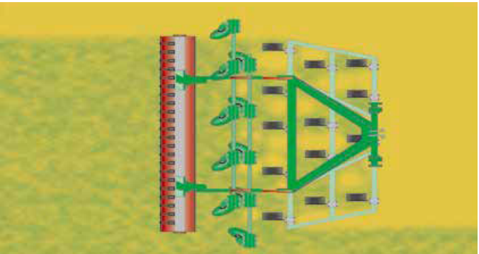
Stroheinarbeitung mit zweibalkigem (Standard-)Flügelchargrubber (oben) und mehrbalkigem Grubber. Quelle: Amazone
